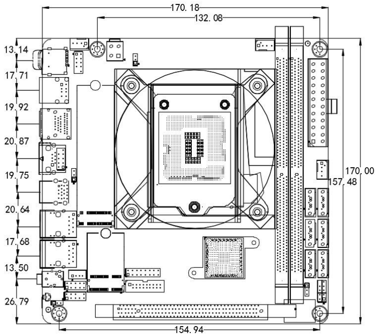
H270S6 VER:01.0 尺寸图
