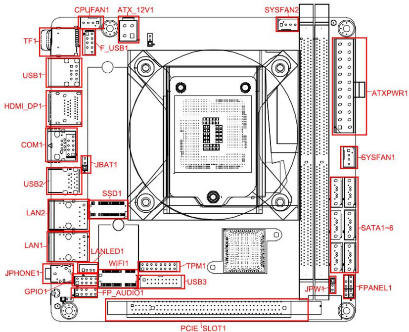
H270S6 VER:1.0 接口位置图
